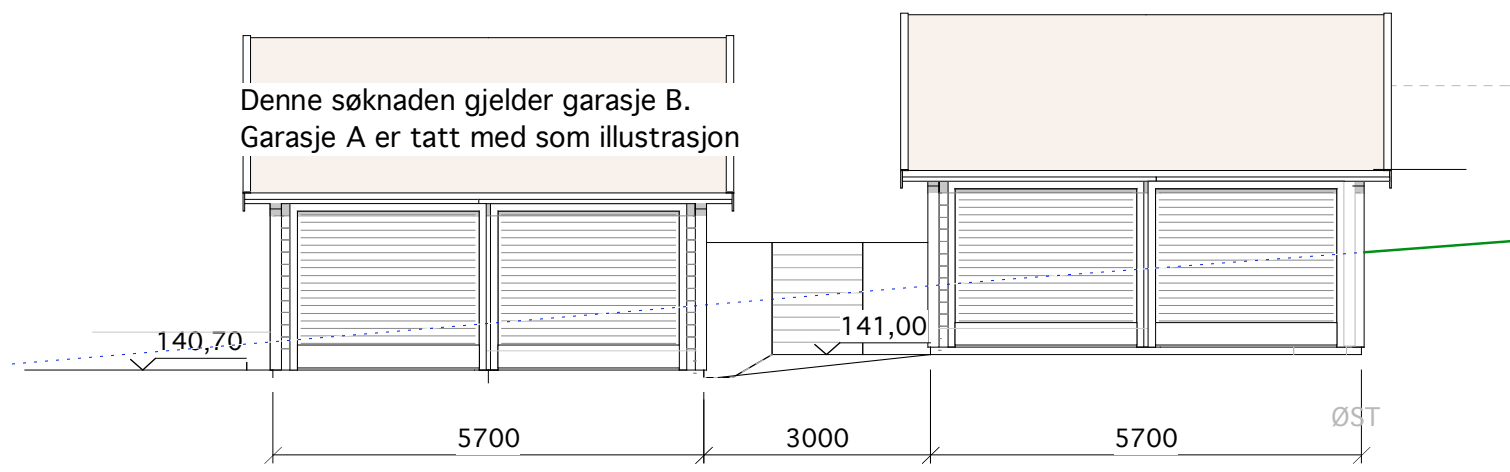
ØST Garasje B
