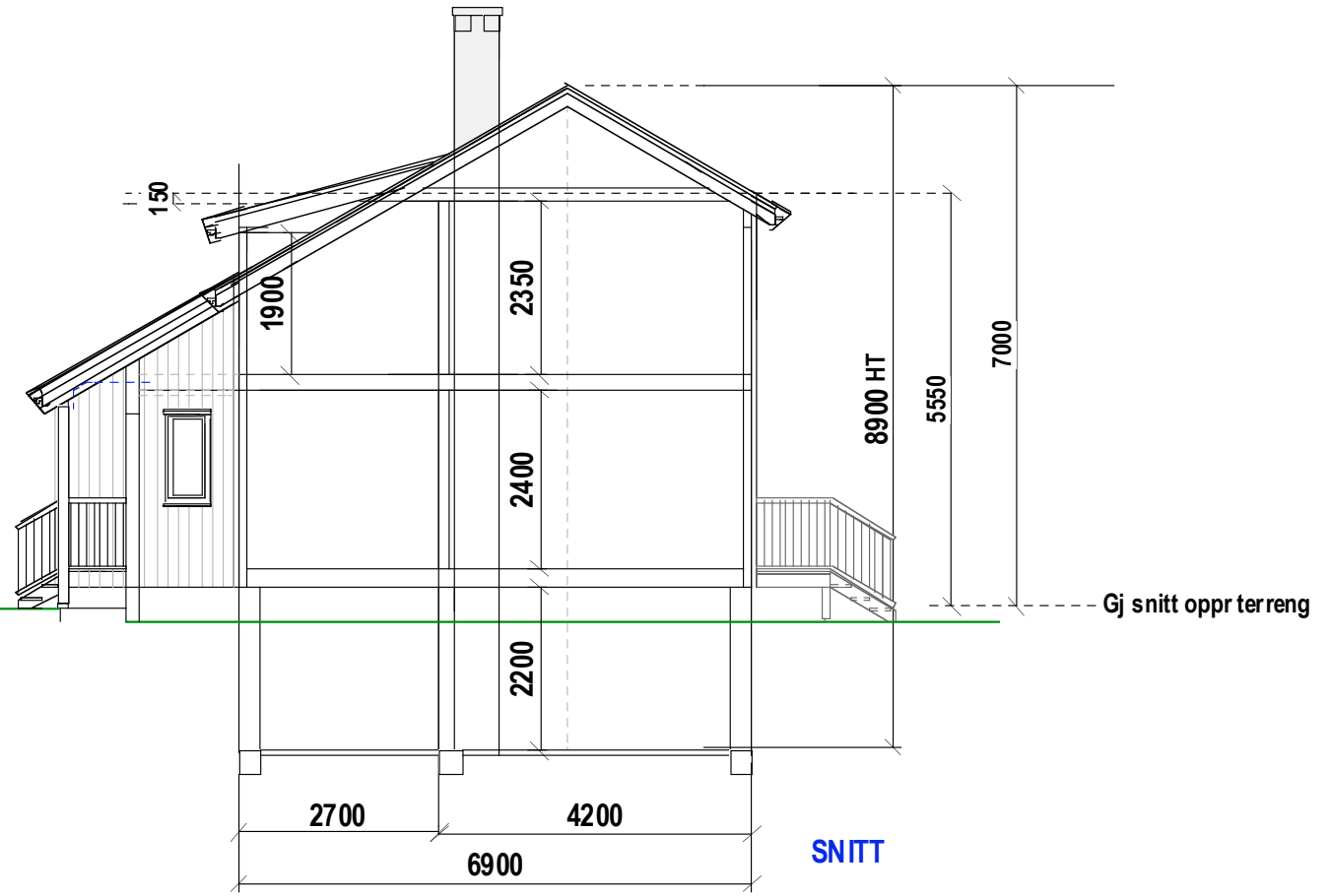
SNITT B-B
