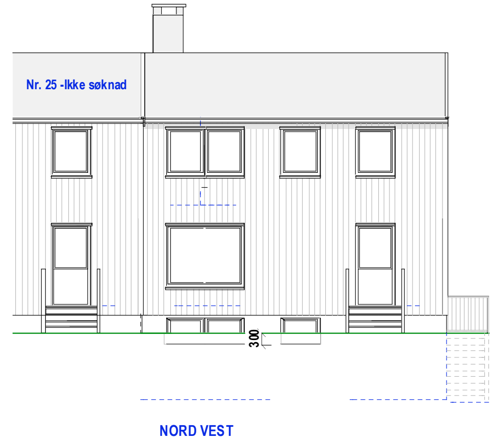
E 1-2- Fasader
