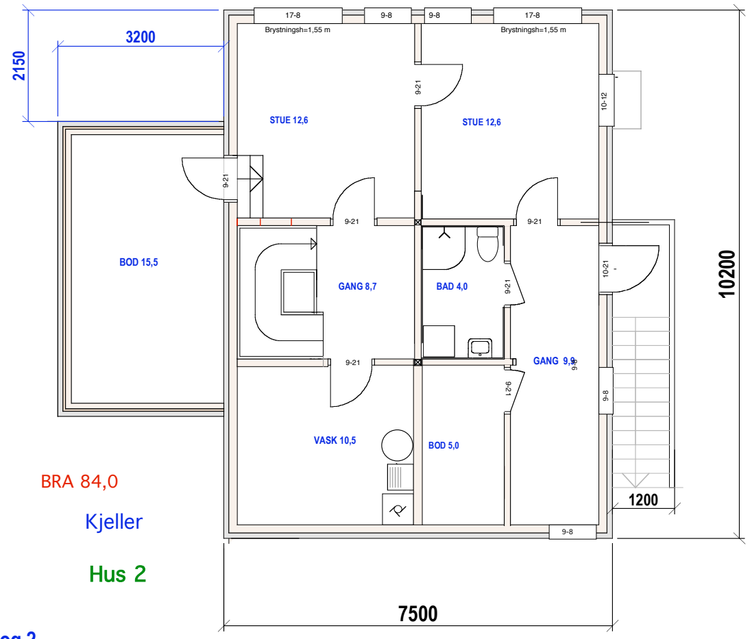
Hus 1 og 2 E.1-2 Plan 1.etg. og kjeller
