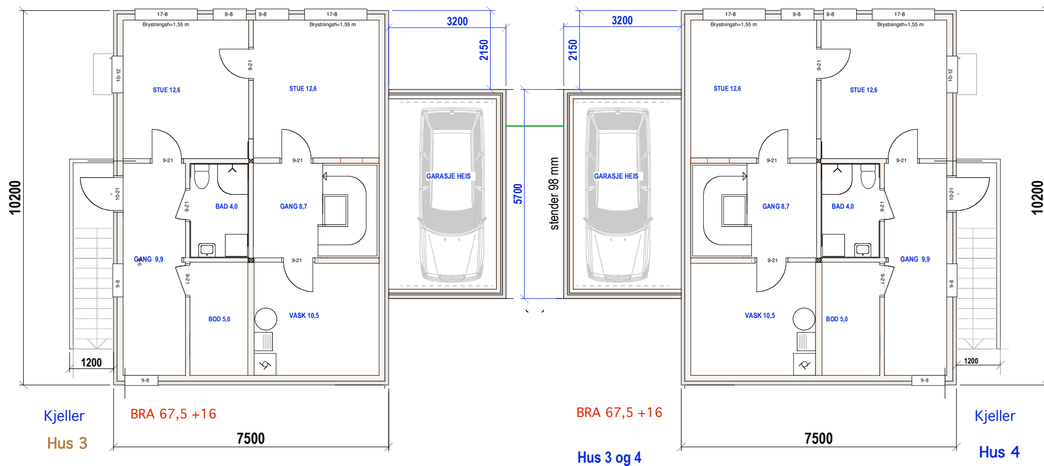
E.1-2 Plan 1. eg og kjeller
