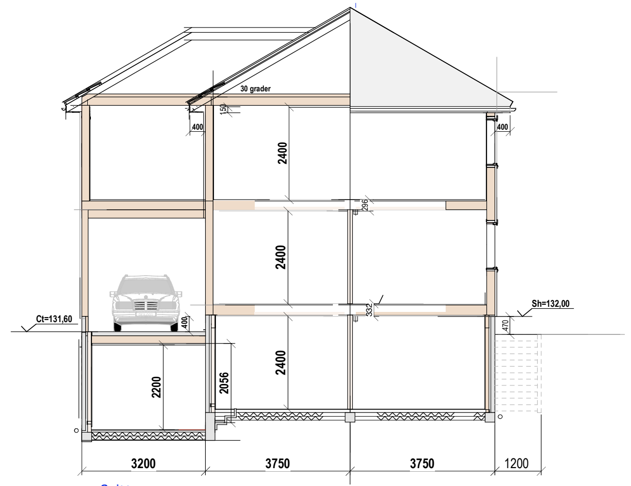
Snitt Hus 2
