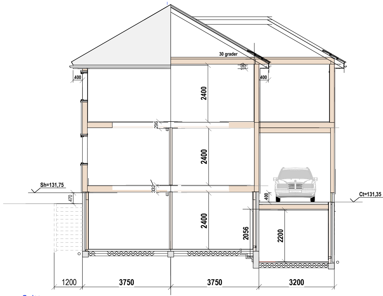
Snitt Hus 1
