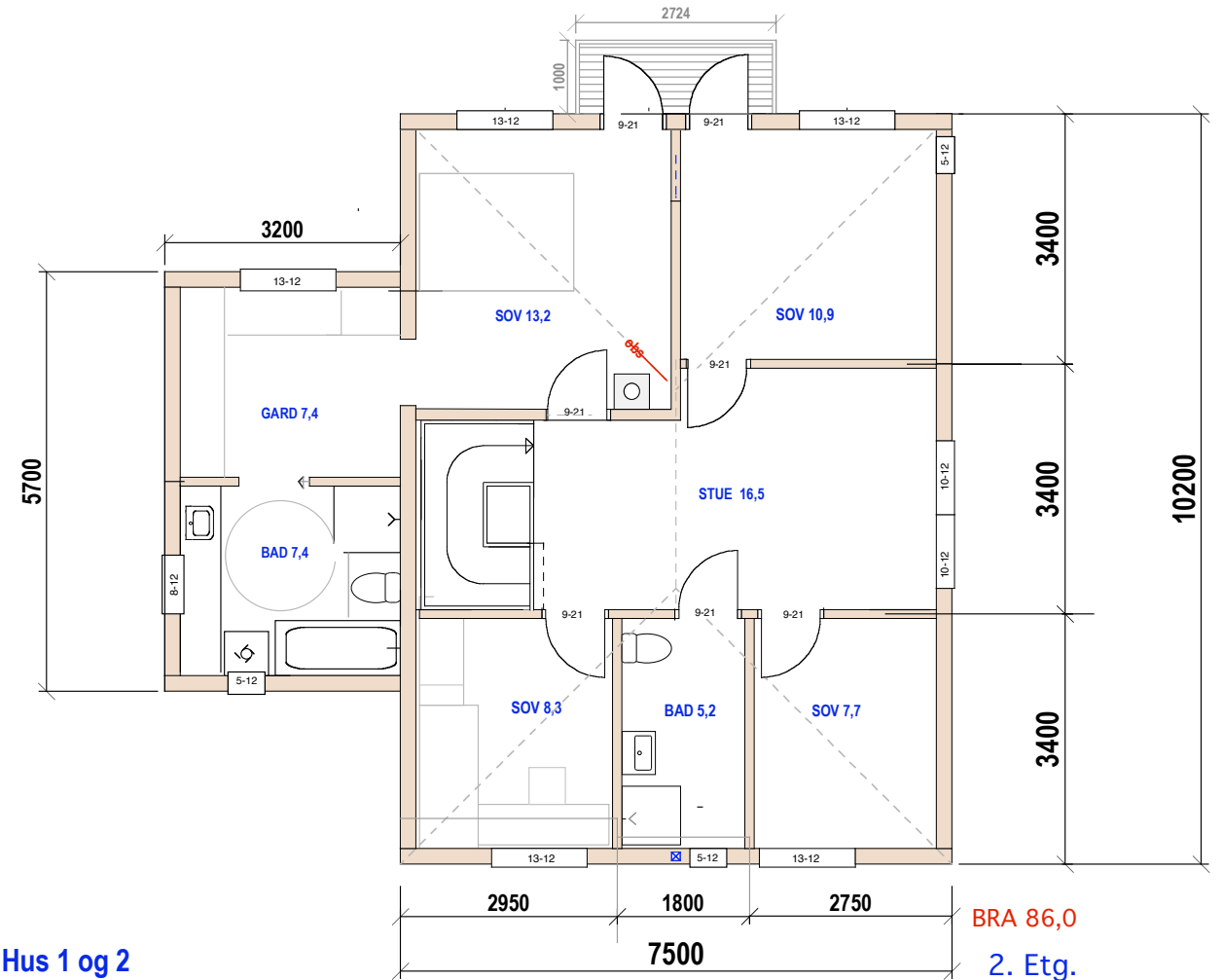
E.1-1 Plan 2. etg og snitt
