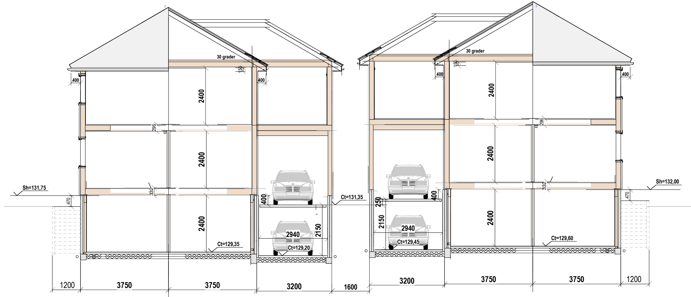
Snittet viser løsning med bilheis
