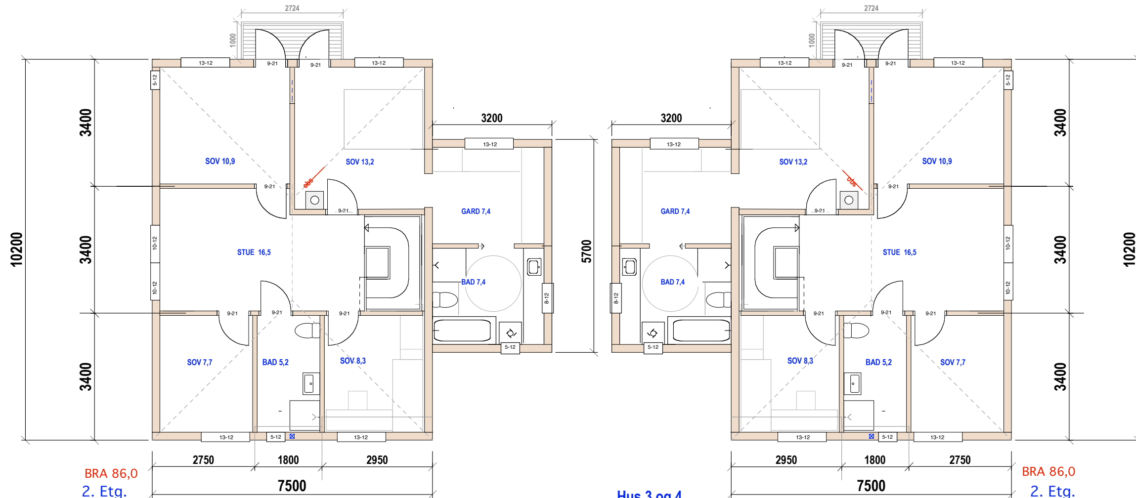
E.1-1 Plan 2. etg og snitt
