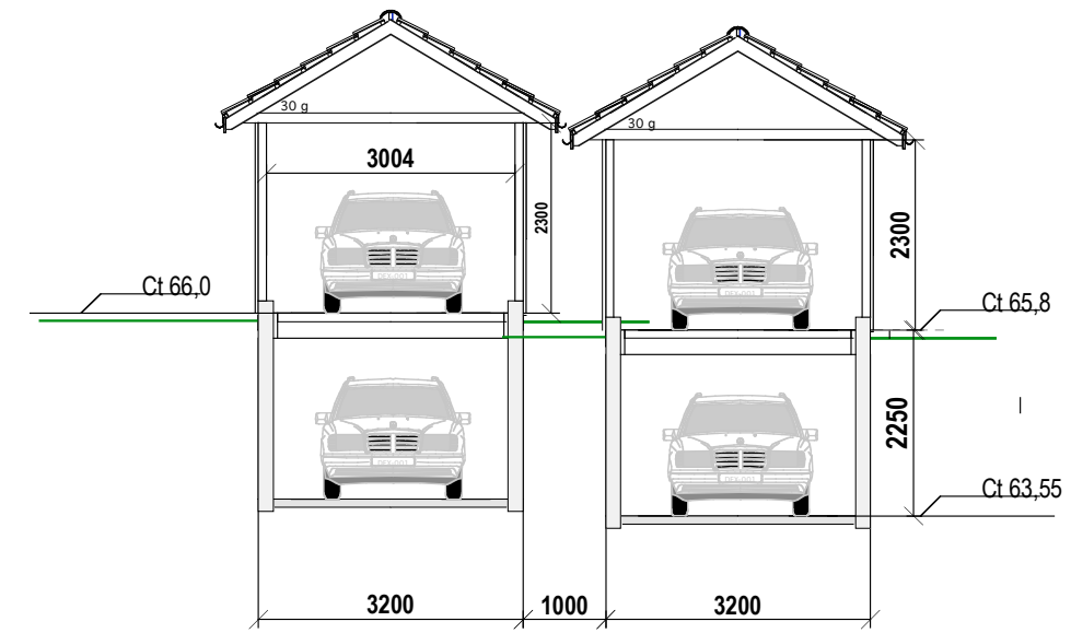
Snitt
