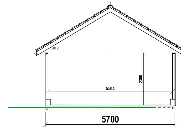
SNITT
