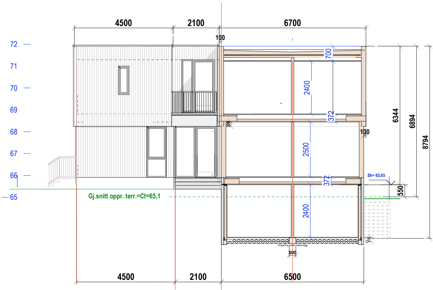
SNITT A-A
