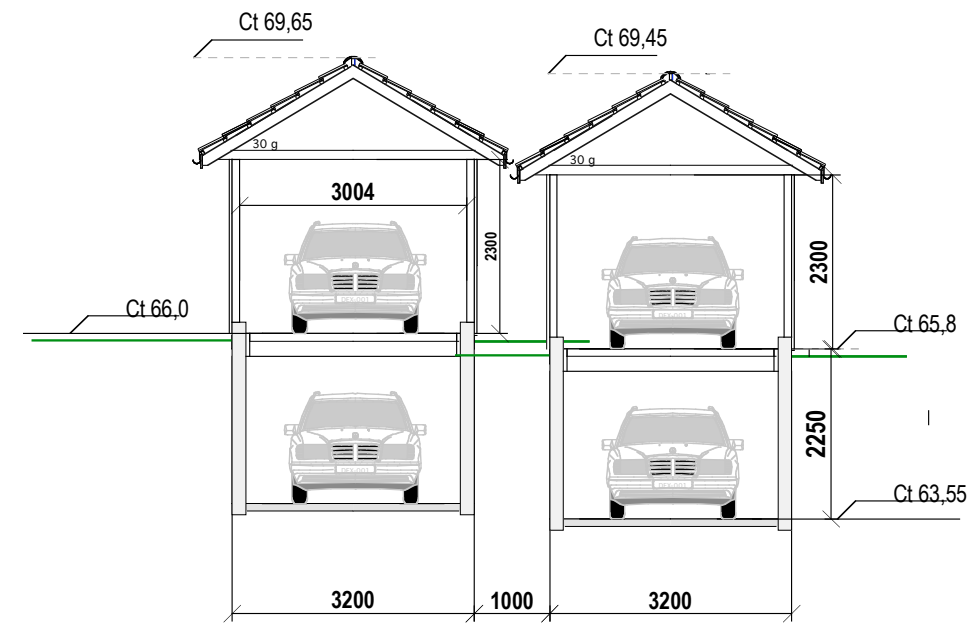
Snitt
