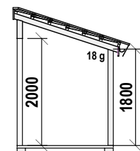
Snitt Bod
