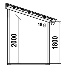
Snitt Leskur
