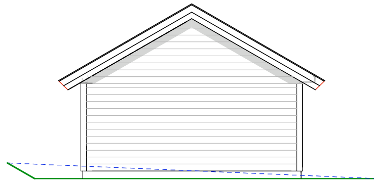
NORD VEST
