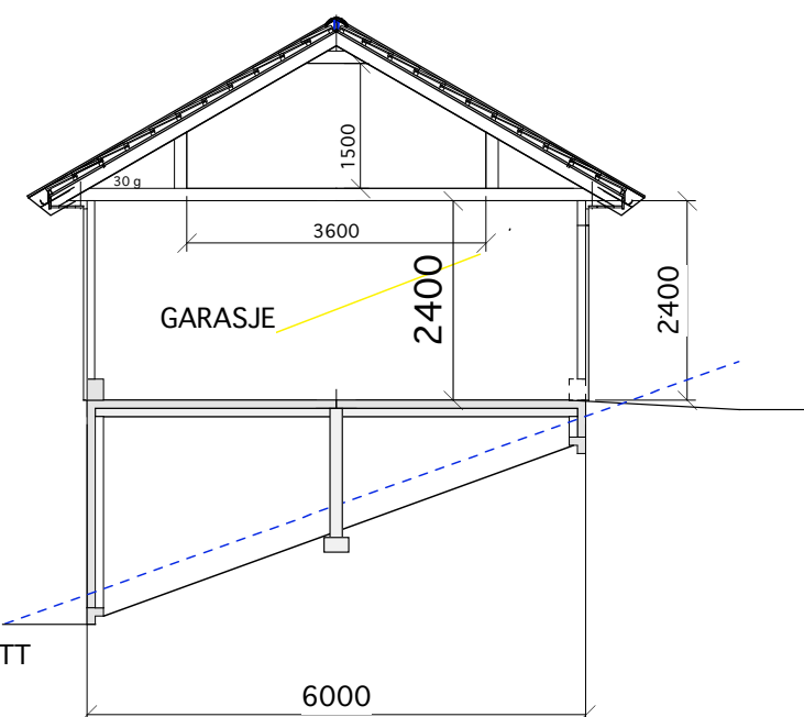
SYD VEST
