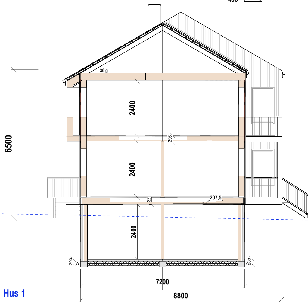
Hus 1 SNITT I GARASJE
