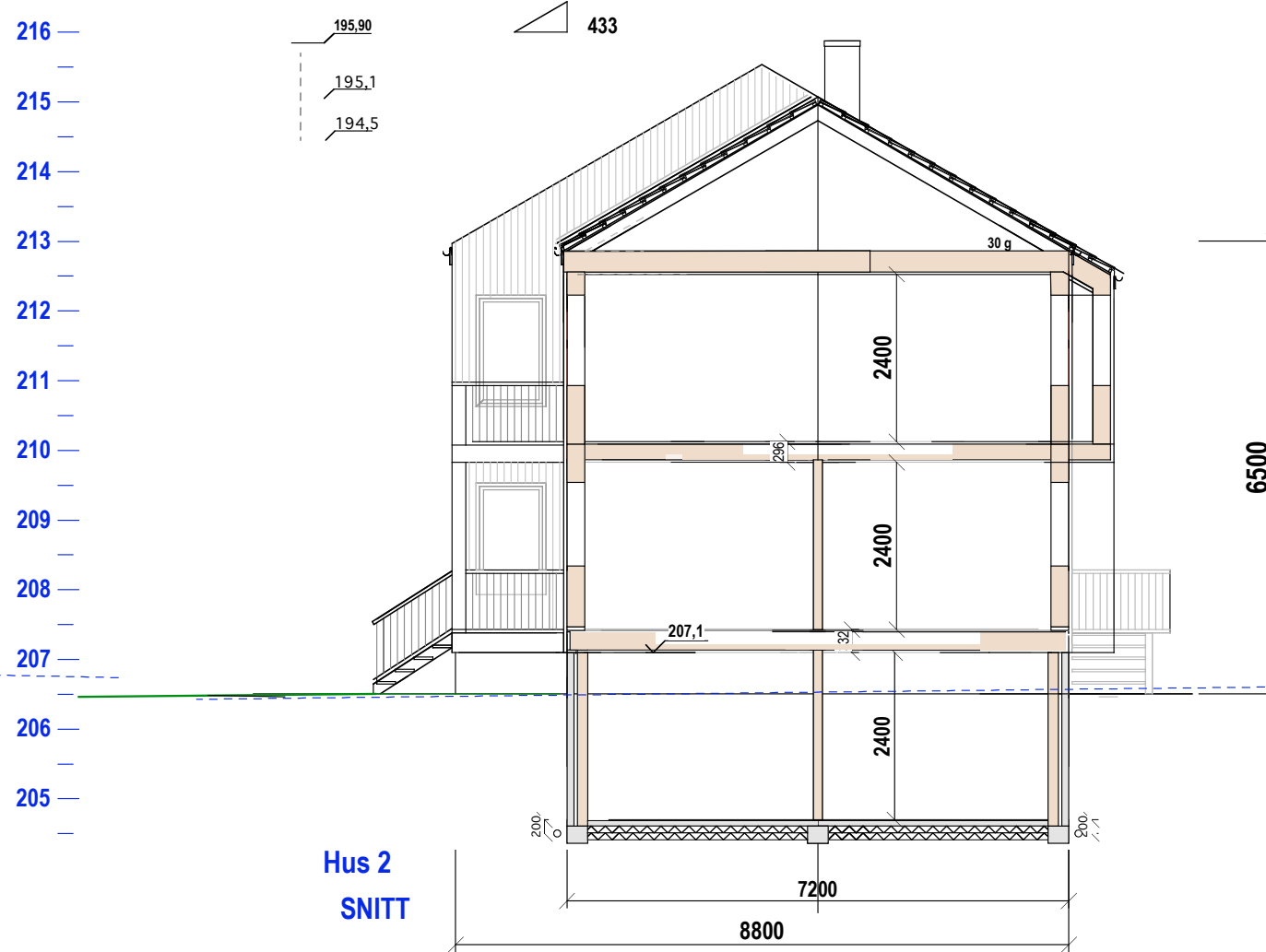
Hus 2 SNITT I GARASJE
