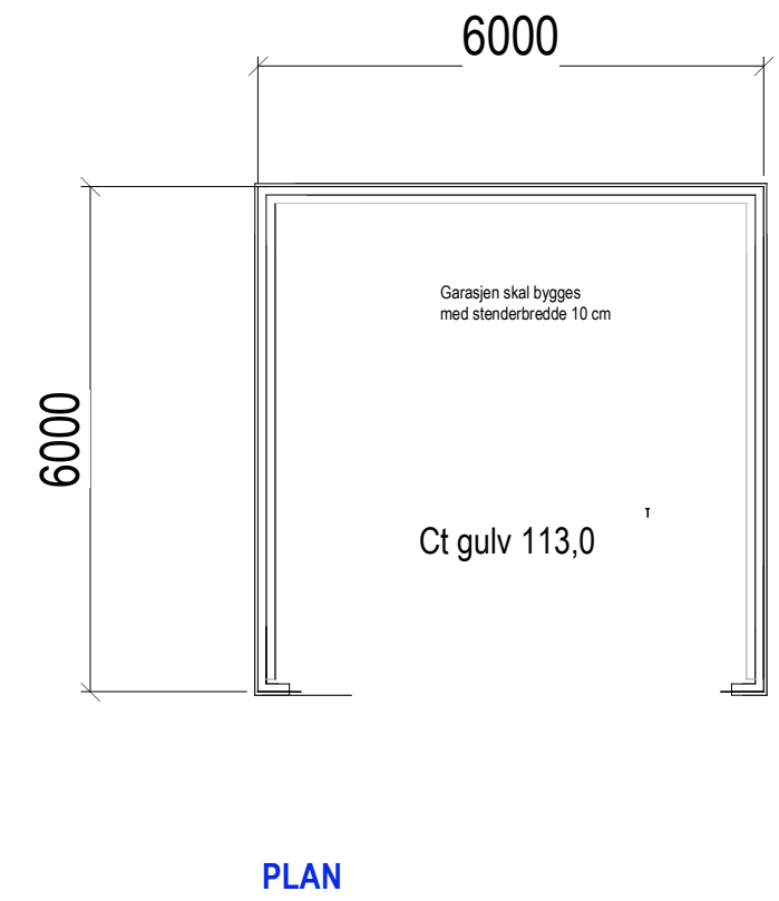
Garasje 1 E.1- Plan, snitt og fasader
