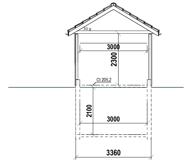
Snitt
