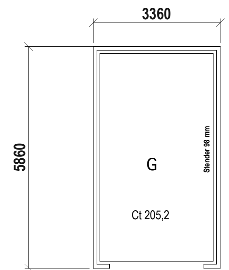
Plan 1.etg
