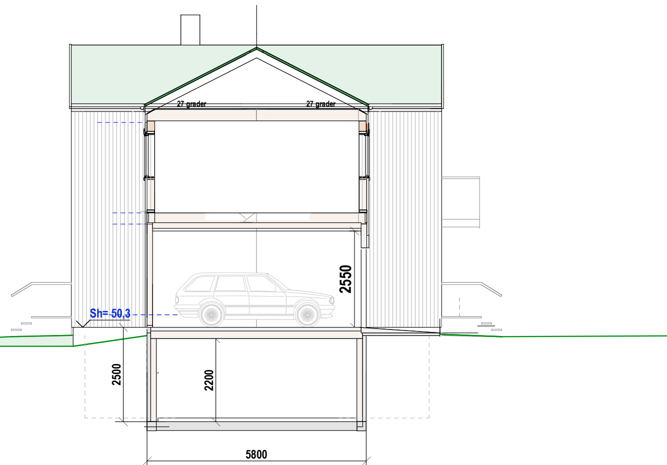
HUS 1-3 Snitt i garasje
