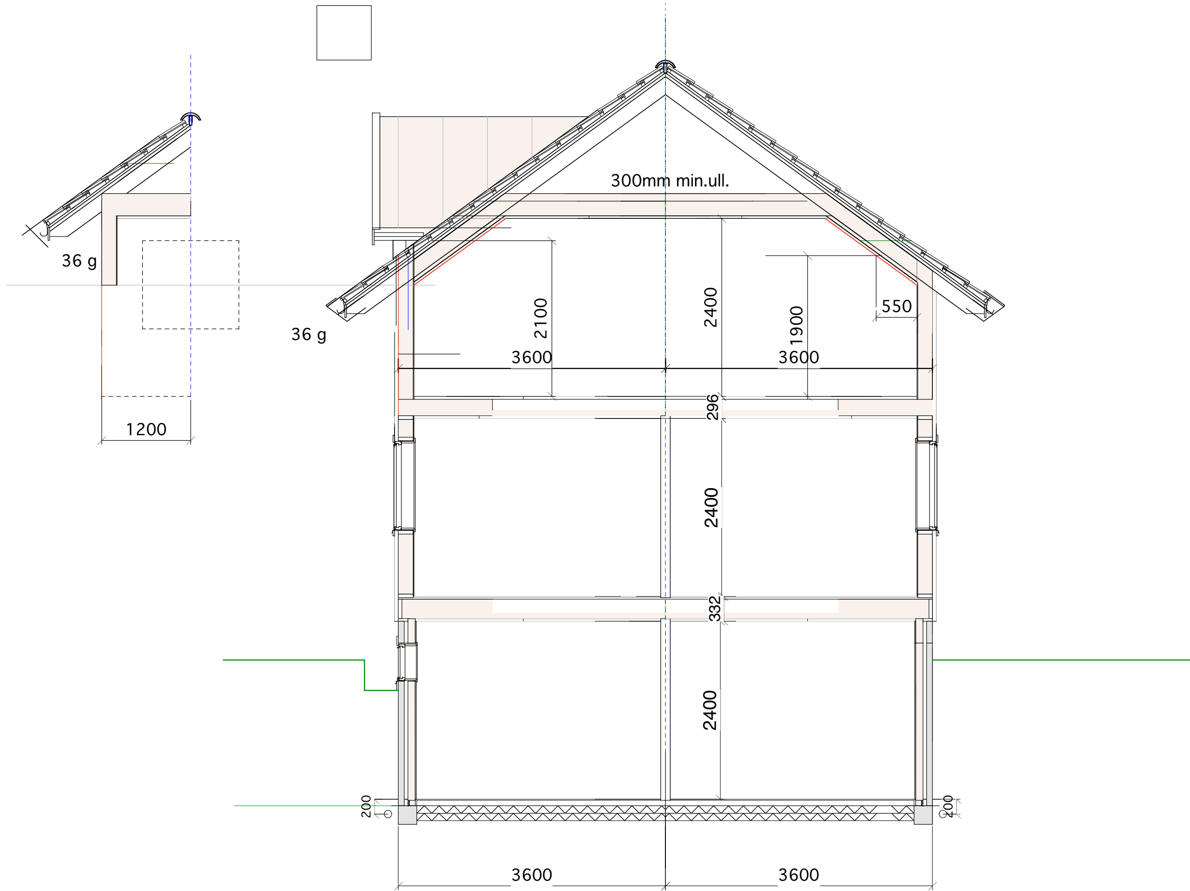
Snitt
