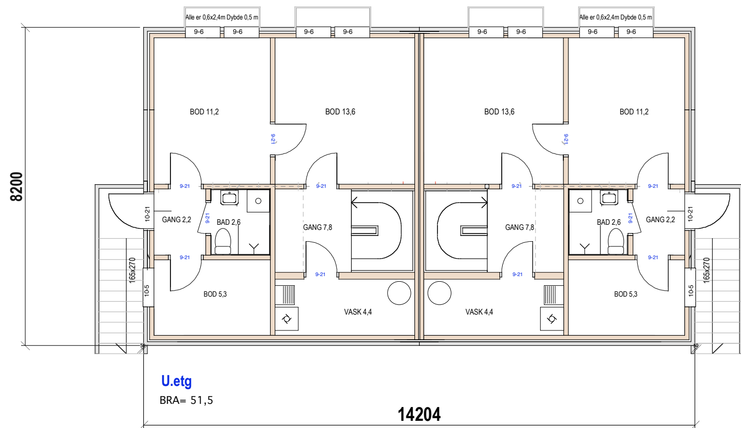
E.1-2 Plan 1.etg og kjeller
